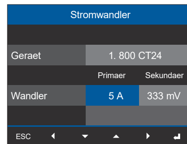
Abb. Fenster Stromwandler - 1. Modul 800-CT24 -> Eintrag Primär für LP-Stromwandler
