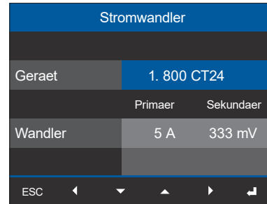
Abb. Fenster Stromwandler 1. Modul 800-CT24 -> Eintrag Gerät
