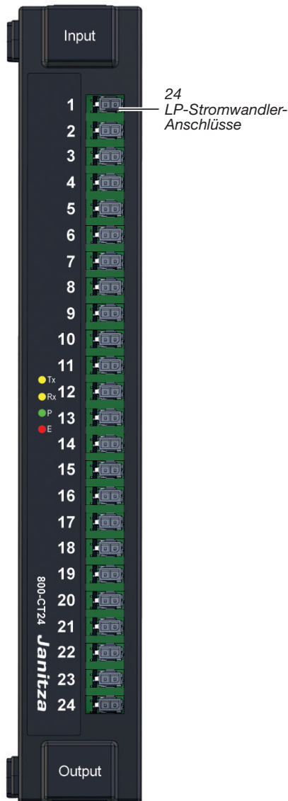
Abb.: Modul 800-CT24
